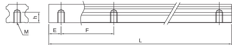
图 2.4.1 下锁式滑轨尺寸图
