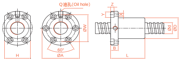
SFNI/SFI 精密研磨级系列规格尺寸表
