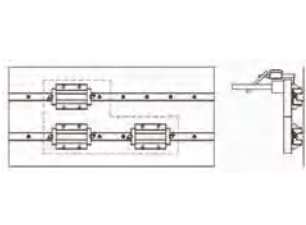
图 1.11.15 移动工作台的方法
