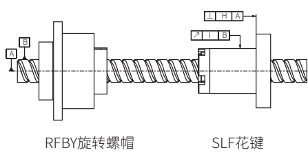
图 1.2.2 RBLY 系列
