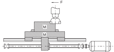
图 1.5.1 负荷惯性矩
