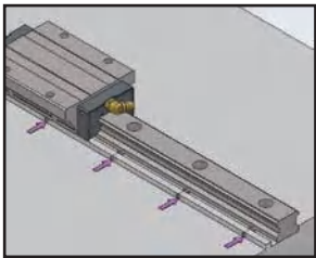
图 1.11.9 安装的检查
