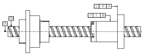
RFSY旋转螺帽
