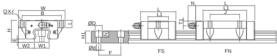
SRS-F 低组装系列规格尺寸表
