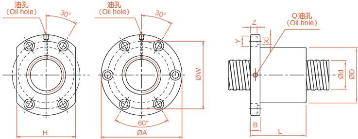
SFV 精密研磨级系列规格尺寸表
