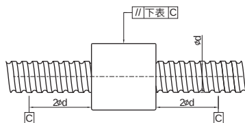
图 1.3.2 方形螺帽平行精度
