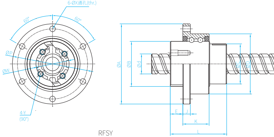
RSSY 精密滚珠螺杆花键规格尺寸表
