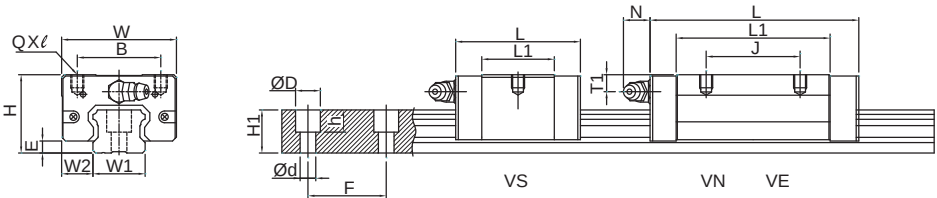
SRS-V 低组装系列规格尺寸表
