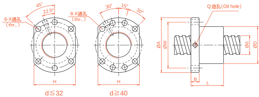
SFNU/SFU (DIN 69051 FORM B) 精密研磨级系列规格尺寸表
