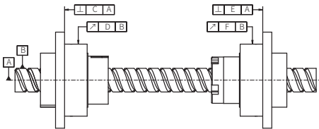
RFSY旋转螺帽
