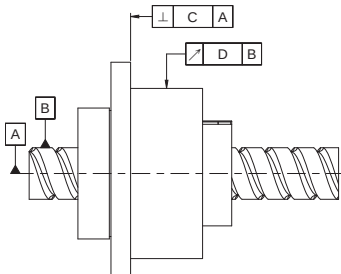
图 1.2.3 RFBY 系列
