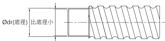
图 1.10.4 出牙—内循环轴端必要条件
