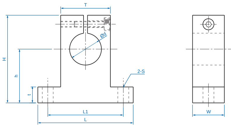
SS 系列规格尺寸表 ( 心轴支撑座 )
