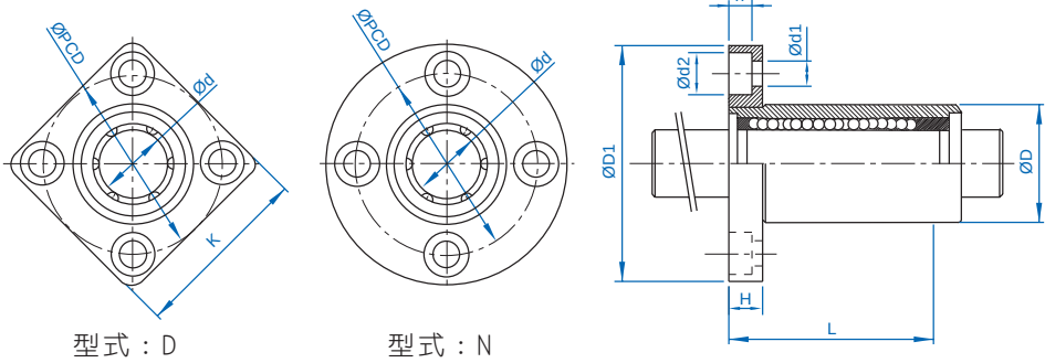
LF-L 系列规格尺寸表 ( 法兰式加长型 )
