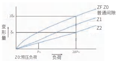
图 1.10.2 刚性数据
