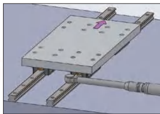
图 1.11.16 仿效基准侧轨道的方法
