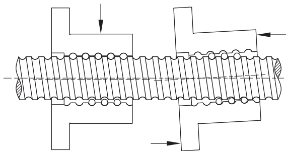
图 1.10.3 偏荷重
