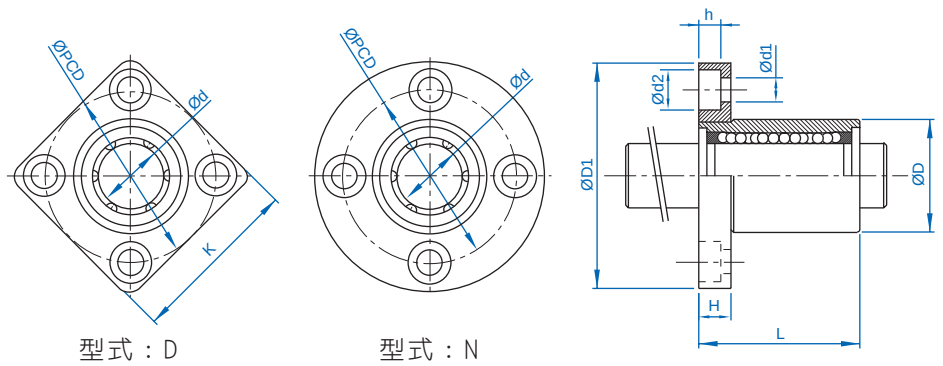
LF 系列规格尺寸表 ( 法兰式 )
