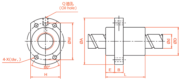
SFY 精密研磨级系列规格尺寸表
