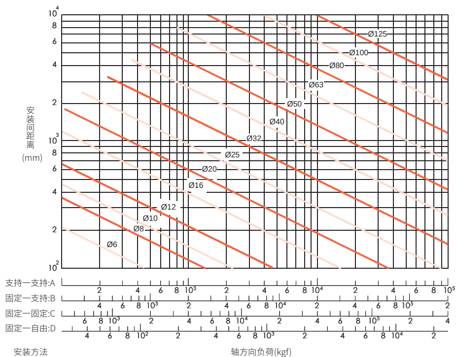
图 1.4.16 屈曲之容许压缩负荷
