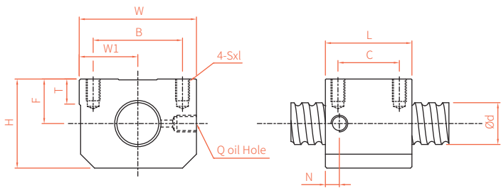
SFSQ 精密研磨级系列规格尺寸表
