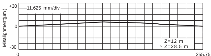
图 1.9.4 工作台的水平变位
