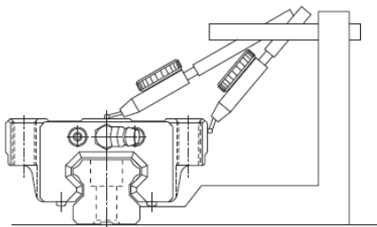
图 1.9.1 行走平行度
