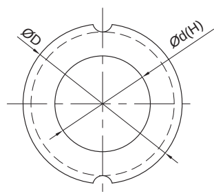
空心花键轴
