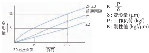
图 1.10.2 刚性数据
